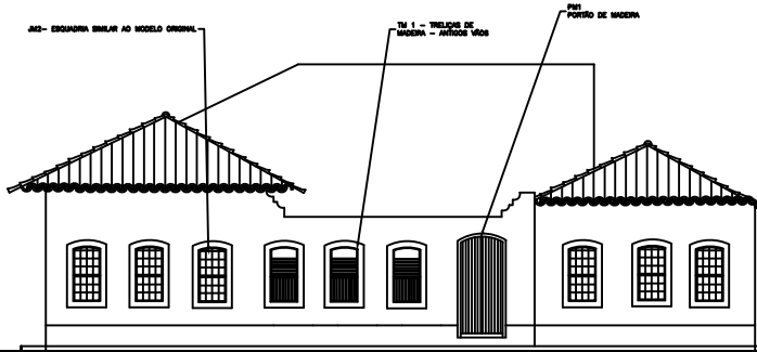
3 - FACHADA POSTERIOR (RUA EXPEDICIONÁRIOS BRASILEIROS)
