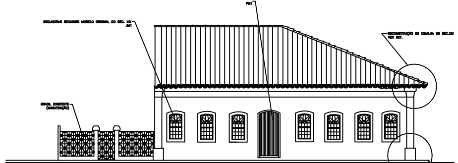
1 - FACHADA FRONTAL (AV. DR. ALTINO ARANTES)
